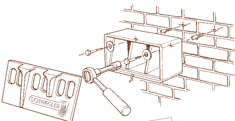
Uniwersalna letnia kwatery dla nietoperzy 2FTH Nr kat. 00 772/8
